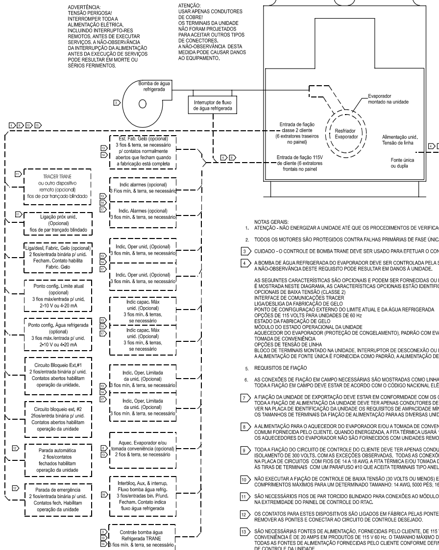
Fig 19 - Layout de Campo, Unidades com 2 Compressores
