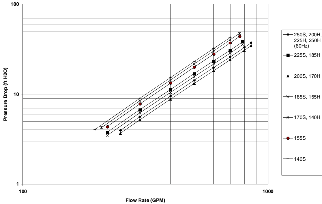
Fig. 11 - Queda de pressão de água no Evaporador, 3 compressores
