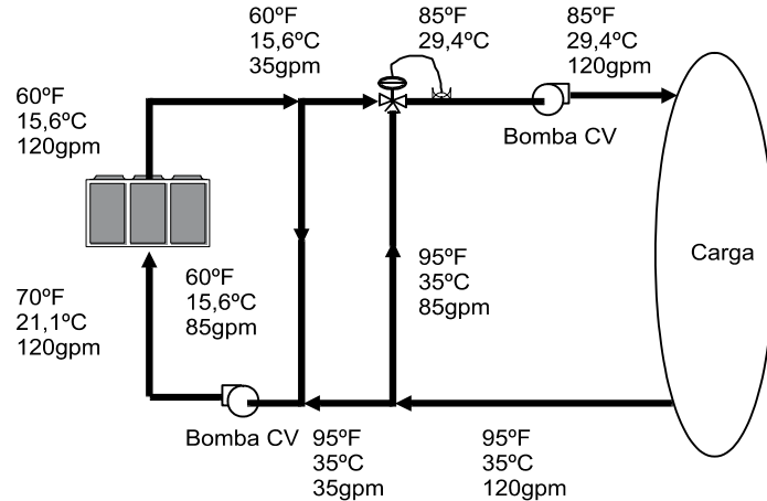
Fig. 06 - Layout do sistema com temperatura fora da faixa
