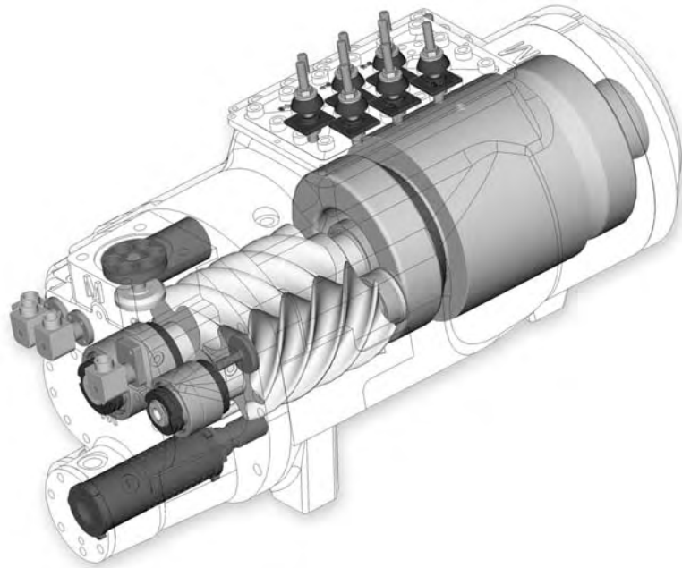
Fig. 02 - Corte de um compressor
