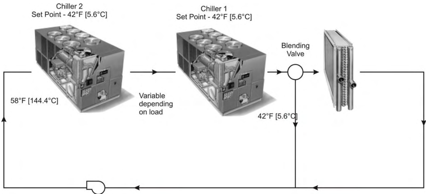
Fig. 07 - Recomendações para a tubulação de água
